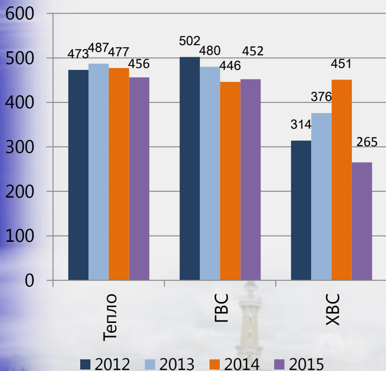
КОЛИЧЕСТВО ПОВРЕЖДЕНИЙ НА СЕТЯХ
