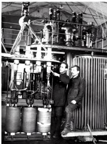
Ремонт трансформатора на электростанции г. Костромы
