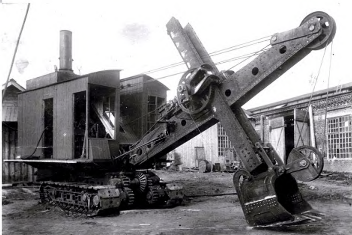
Первая продукция завода «Рабочий металлист» – паровой экскаватор
