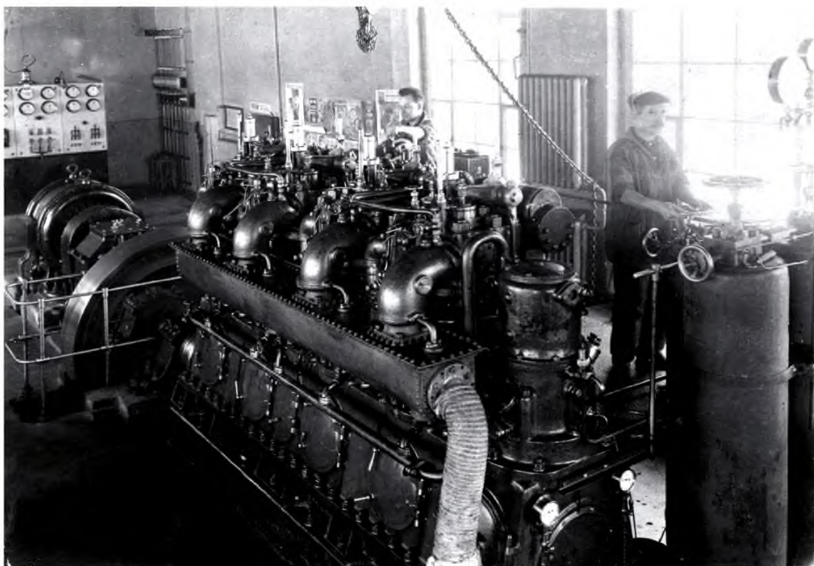
Машинное отделение обувной фабрики «X Октябрь». 20 марта 1936 г.
