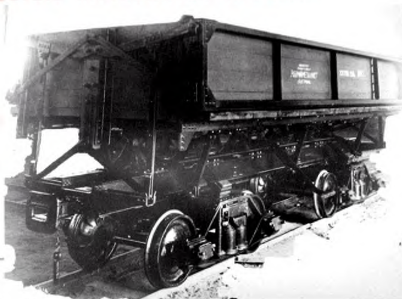
Вагонетка с опрокидывающейся платформой
