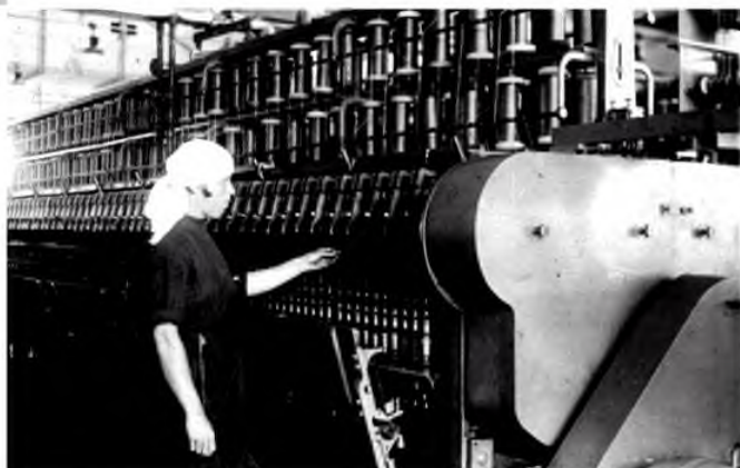
В ватерном цехе комбината системы инженера И.Д. Зворыкина
