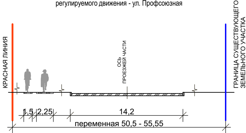
Поперечный профиль 1-1 Существующая магистральная улица общегородского значения регулируемого движения - ул. Профсоюзная
