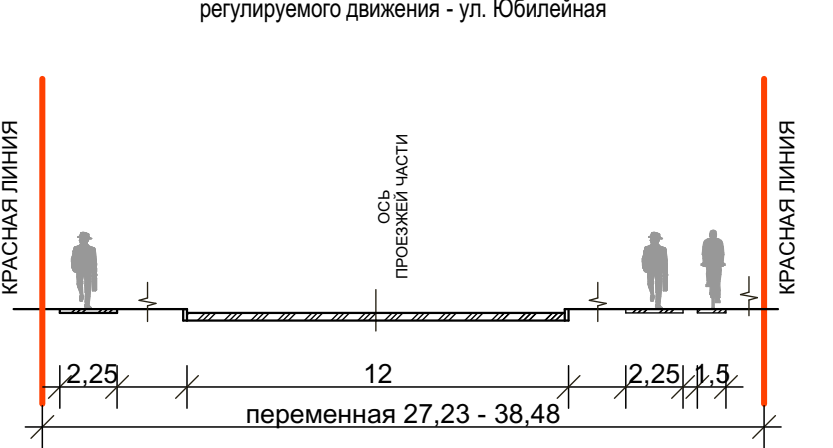
Поперечный профиль 2-2 Существующая магистральная улица общегородского значения регулируемого движения - ул. Юбилейная
