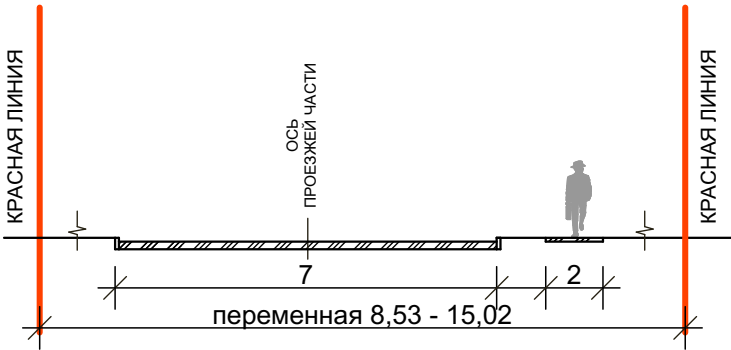
Поперечный профиль 4-4 Существующая улица местного значения
