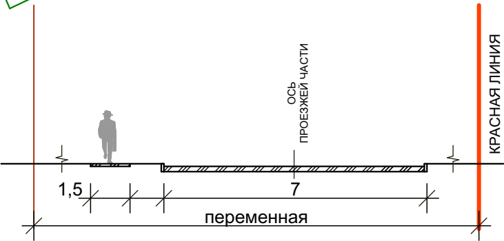
Поперечный профиль 3-3 Существующая улица местного значения
