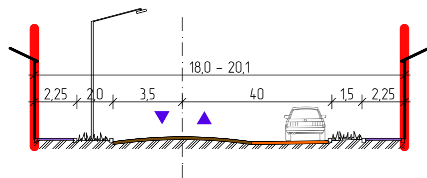
Поперечный профиль улицы 1 Мая
